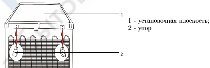
Рисунок Б.1а - Схема крепления упоров к плоскости установочной
